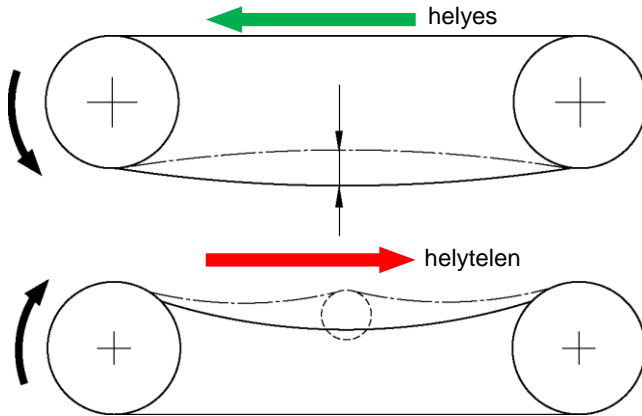
A szállítószalagok futási iránya
