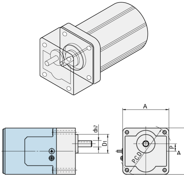
Hajtómotor méretei
