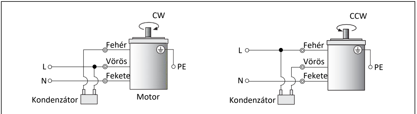
Indukciós motor bekötési ábrája 6W-25W-40W-60W-90W – 230V/50Hz – 1-fázisú
