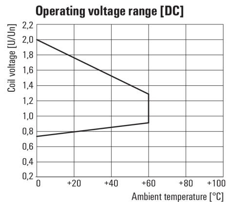
Betriebsspannungsbereich DC
