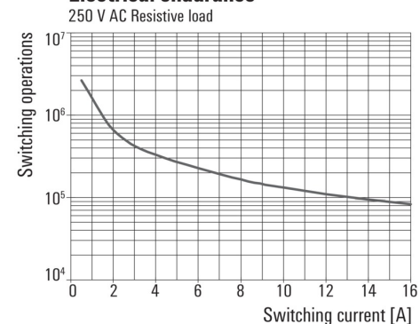
Elektrische Lebensdauer 250 V AC ohmsche Last
