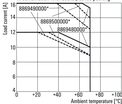
Deratingkurve Relais in Kombination mit Sockel
