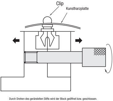
Durch Drehen des gerändelten Stifts wird der Block geöffnet bzw. geschlossen.
