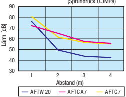
■ Darstellung der Geräuschdaten (Sprühdruk 0.3MPa)
