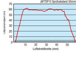
■ Darstellung der Geschwindigkeitsdaten (AFTSP15 Sprühabstand 50mm)
