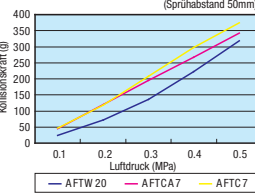
■ Eigenschaften der Luftkollisionskraft Tabelle (Sprühabstand 50mm)
