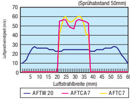
■ Darstellung der Geschwindigkeitsdaten (Sprühabstand 50mm)
