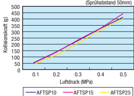
■ Darstellung der Luftkollisionskraftdaten (Sprühabstand 50mm)
