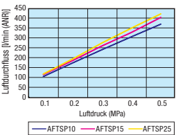
■ Darstellung der Luftdurchflussdaten
