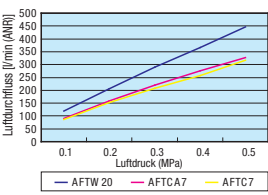
■ Darstellung der Luftdurchflussdaten
