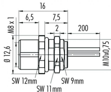
Maßzeichnung
