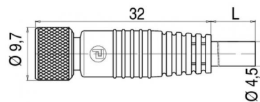
Maßzeichnung
