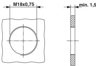
Einbaumaße: ST-17.1N8A6100S, Durchgangsbohrung mit Gewinde (Empfehlung bei Einbau in Stahlblechwand)
