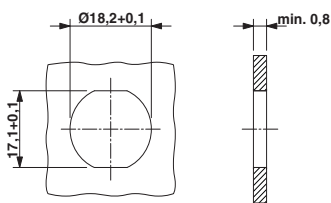
Einbaumaße: ST-.E.1N8A6100S, Bohrung mit Verdreherschutz und Kontermutter (Empfehlung bei Einbau in Stahlblechwand)
