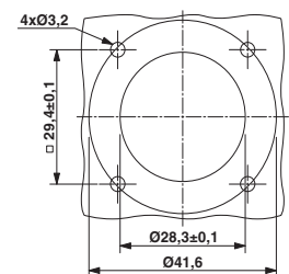
Einbaumaße: SF-EP1N8AC0.., SF-EP1N8ACL..
