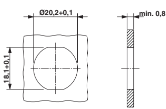
Einbaumaße: ST-.E.1N8AH100S, Bohrung mit Verdreherschutz und Kontermutter (Empfehlung bei Einbau in Stahlblechwand)
