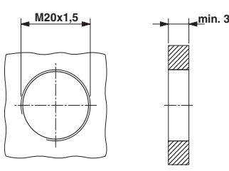
Einbaumaße: ST-17.1N8AH100S, Durchgangsbohrung mit Gewinde (Empfehlung bei Einbau in Stahlblechwand)
