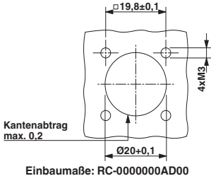
Einbaumaße: RC-0000000AD00
