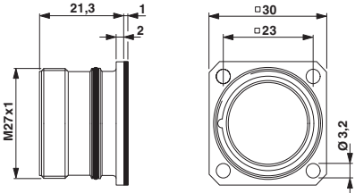
HC-...1N..2300 Flachdichtung
