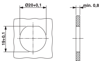
RC-00000006100, Montage Bohrung mit Verdreherschutz und Kontermutter (Empfehlung bei Einbau in Stahlblechwand)
