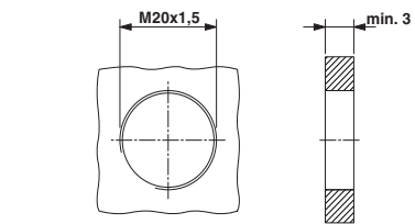
RC-00000006100, Montage Durchgangsbohrung mit Gewinde (Empfehlung bei Einbau in Stahlblechwand)
