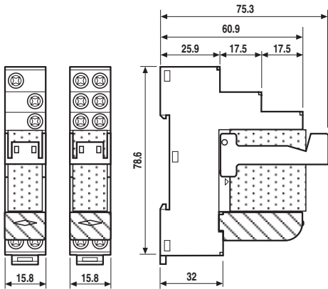
48.31 48.32 / 48.52 / 48.61 / 48.62 Schraubklemmen
