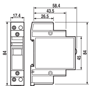
Typ 22.23 Schraubklemmen
