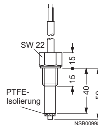
Einpilge Elektrode, stabile Ausführung 3UG32 07-1C
