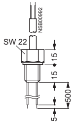
Zweipolige BÜgelelektrode 3UG32 07-2B
