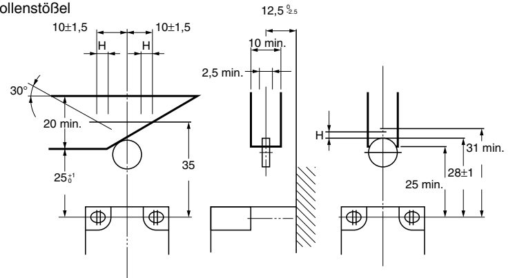
Rollenstößel
