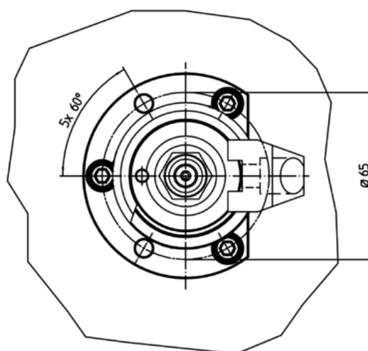
Einbaubeispiel Lochkreis:
