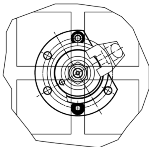
Einbaubeispiel Nutsystem:
