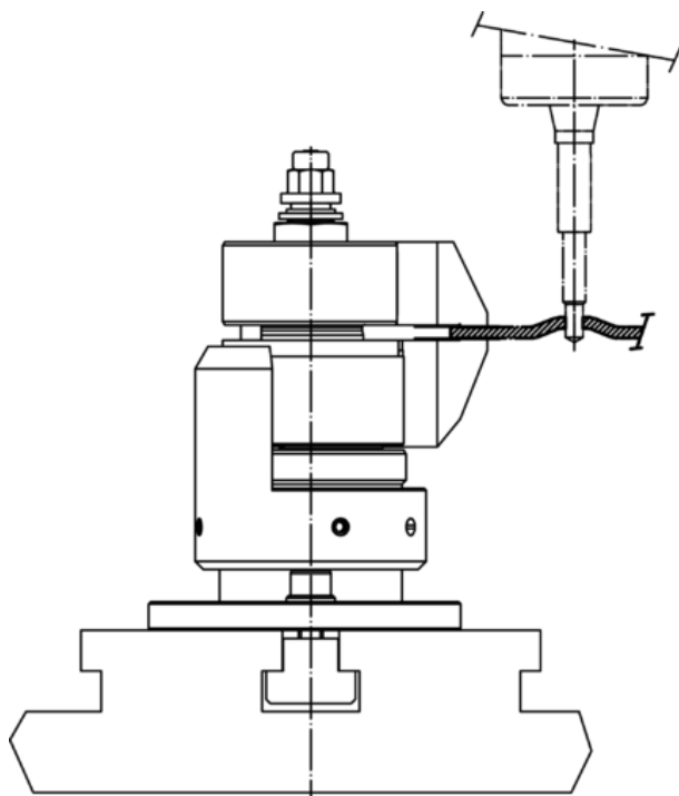
Einbaubeispiel Nutsystem:
